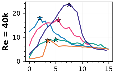
Cl/Cd vs \alpha
