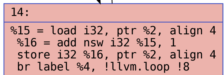
CFG for 'main' function
