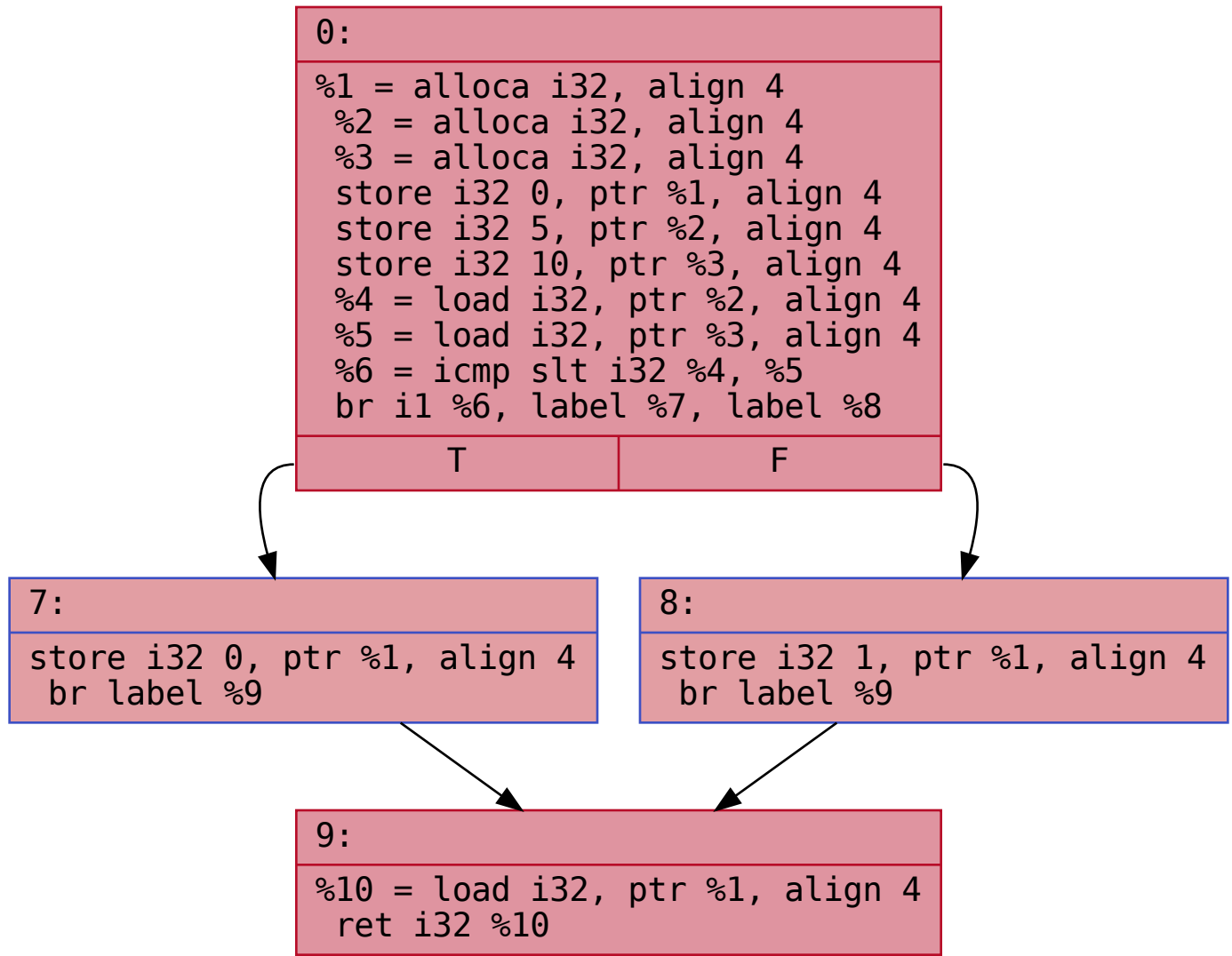
CFG for 'main' function
