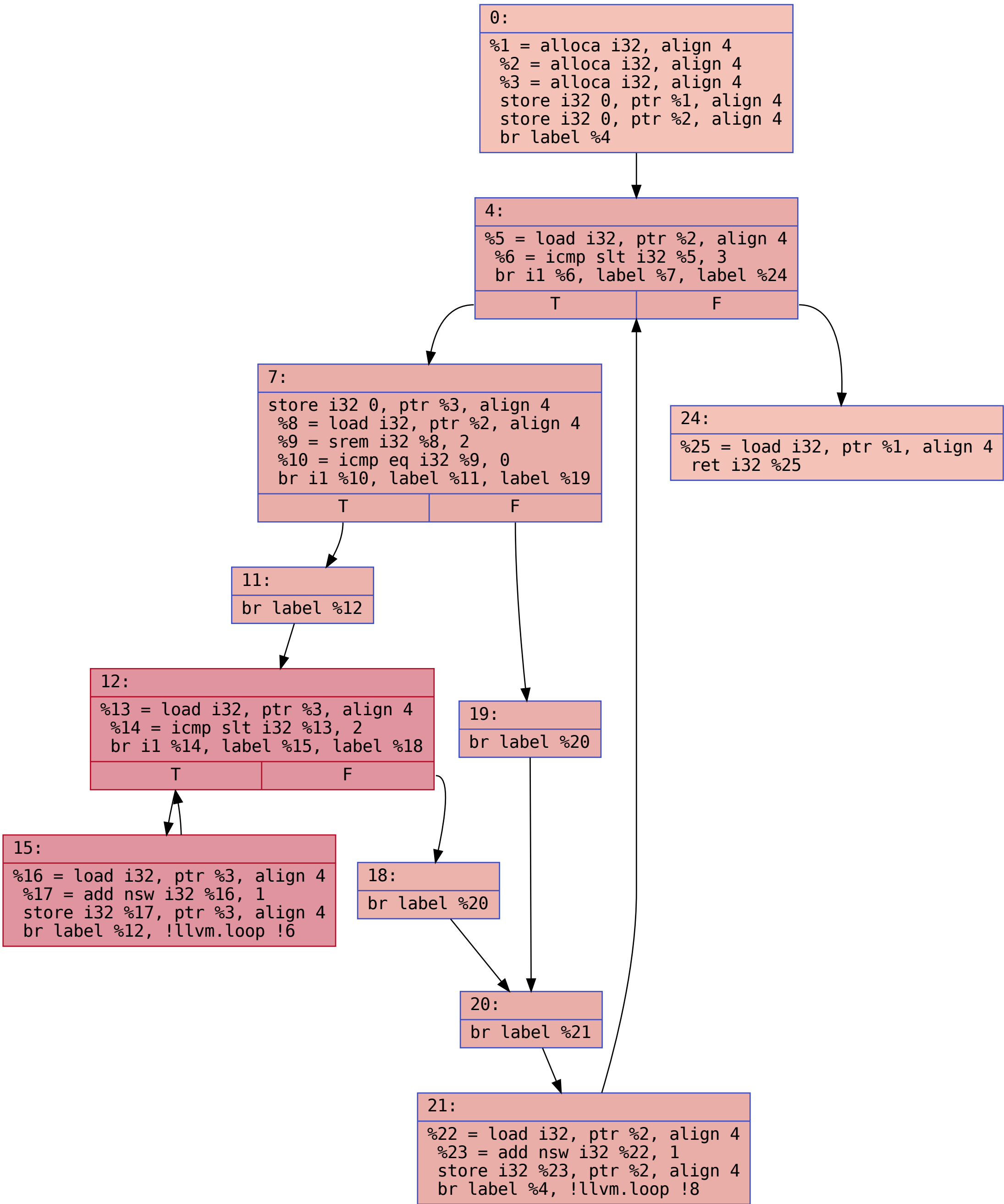
CFG for 'main' function
