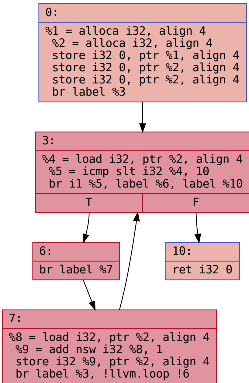
CFG for 'main' function
