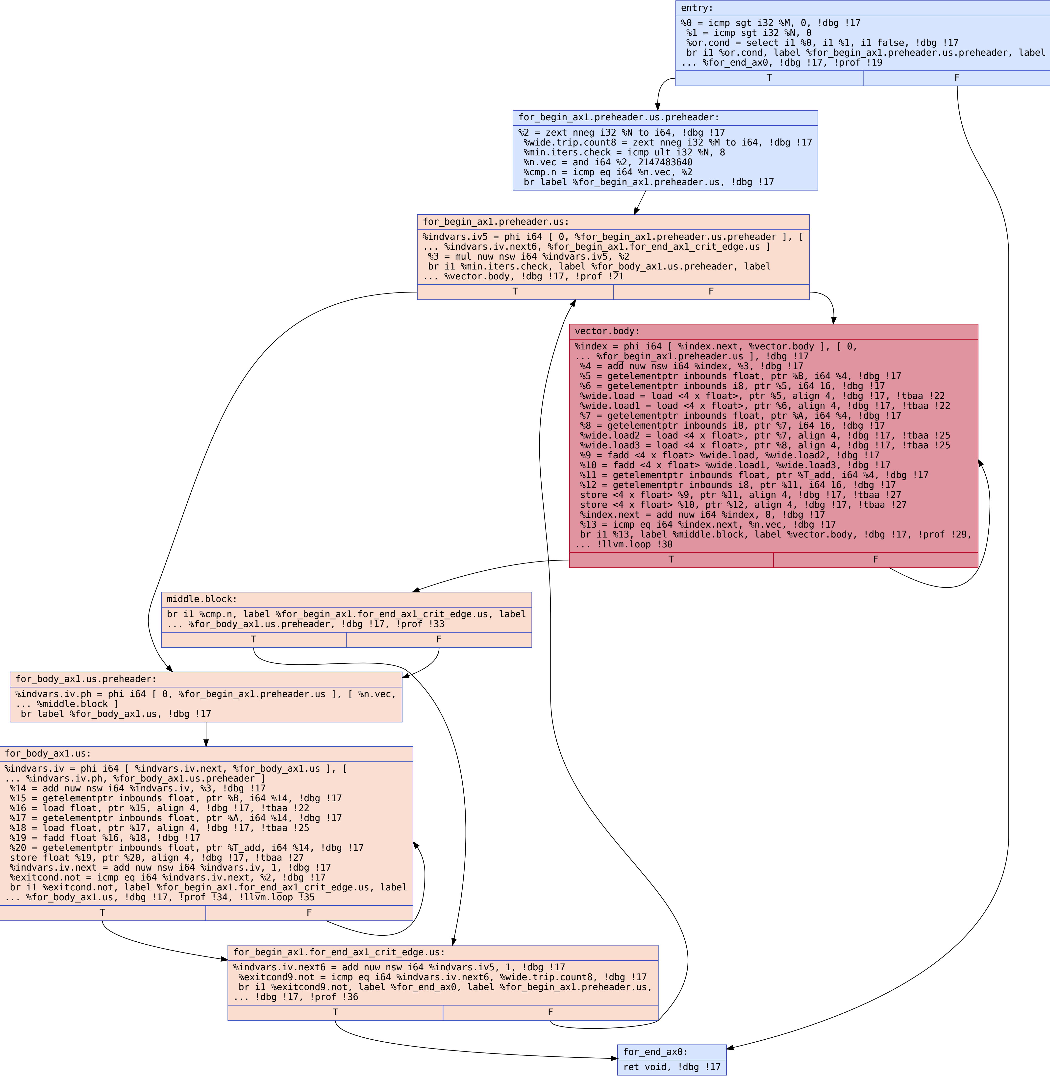
CFG for 'add_compute_' function
