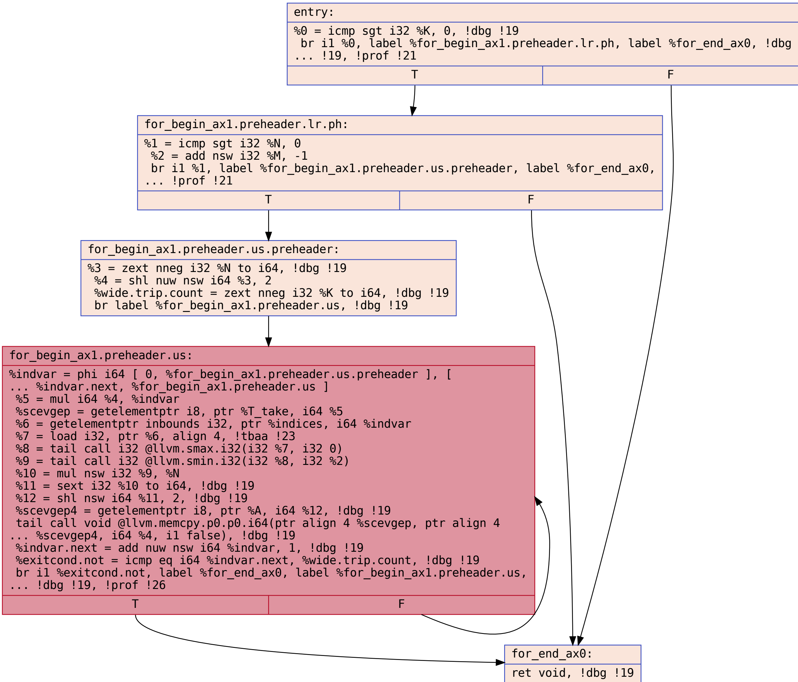
CFG for 'gather_compute_' function
