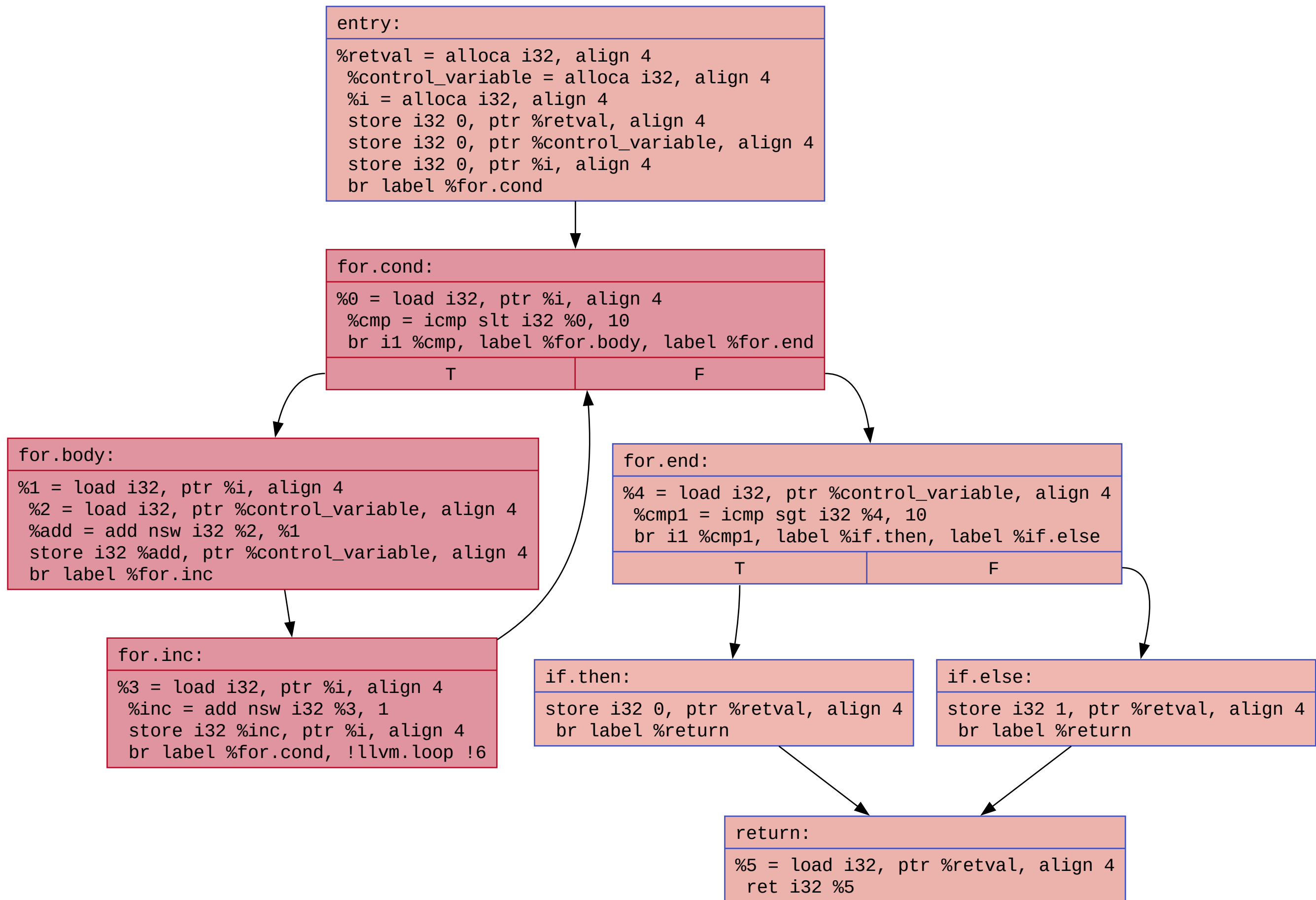
CFG for 'main' function
