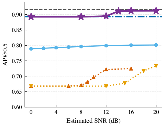
AP@0.5 — AWGN
