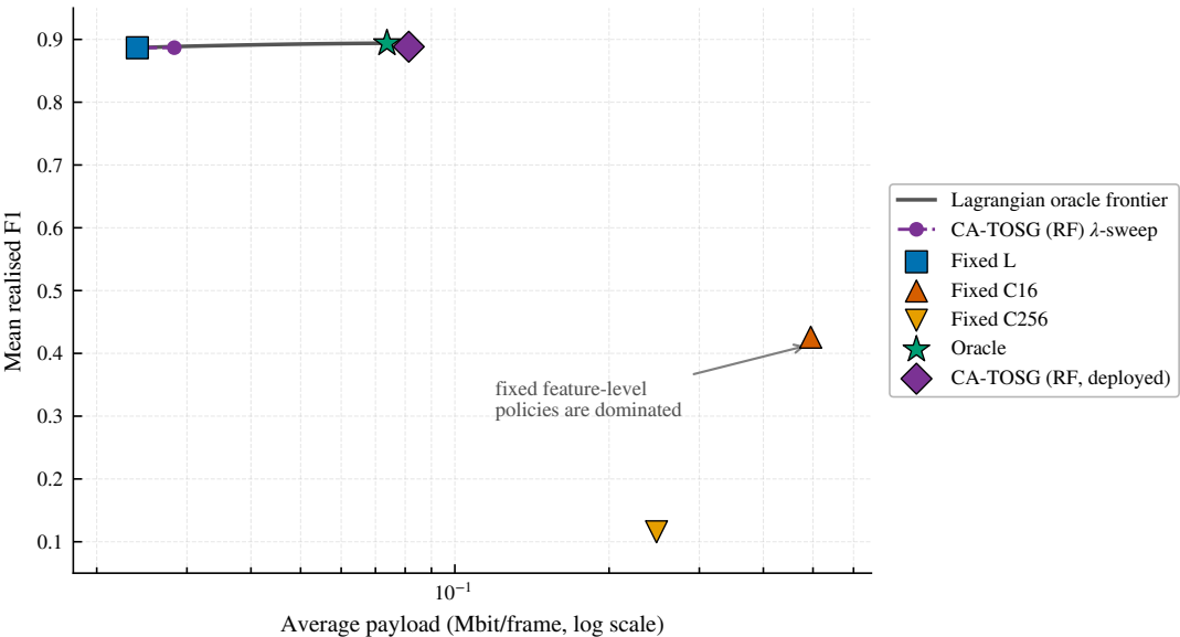
OPV2V test
