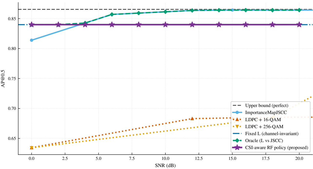
AP@0.5 vs SNR — RAYLEIGH
