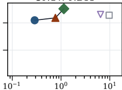
UNSW-NB15
