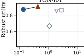
TON-IoT
