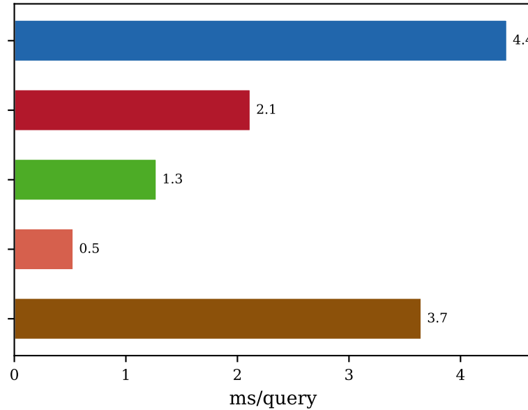
Diginetica
