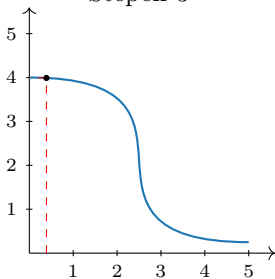
v_I [V] Stepen 3
