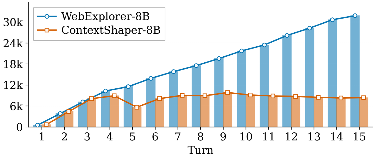
Input Tokens
