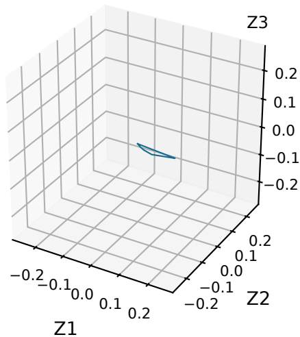
Z_chiral
