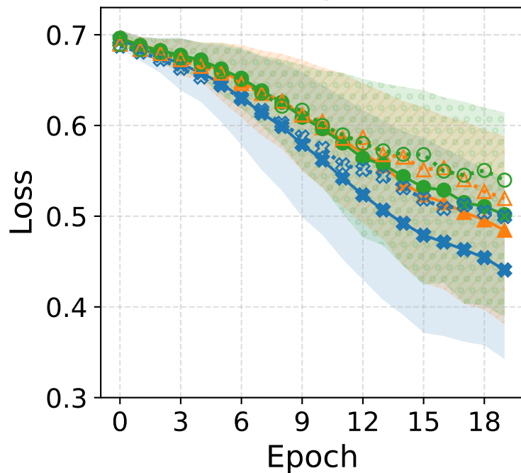
Model: HQCNN-EZ
