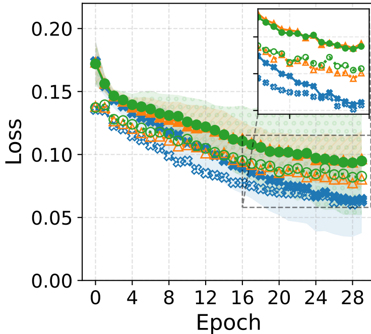
Model: HQCNN-EZ
