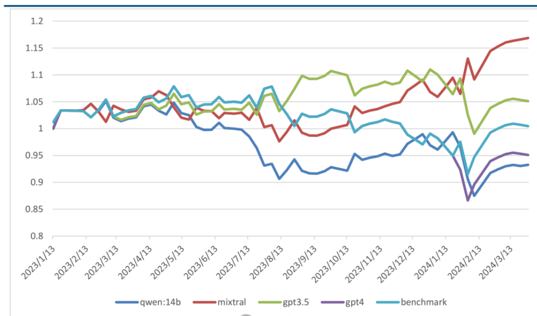
图 16: LLM 上证综指多空择时净值
