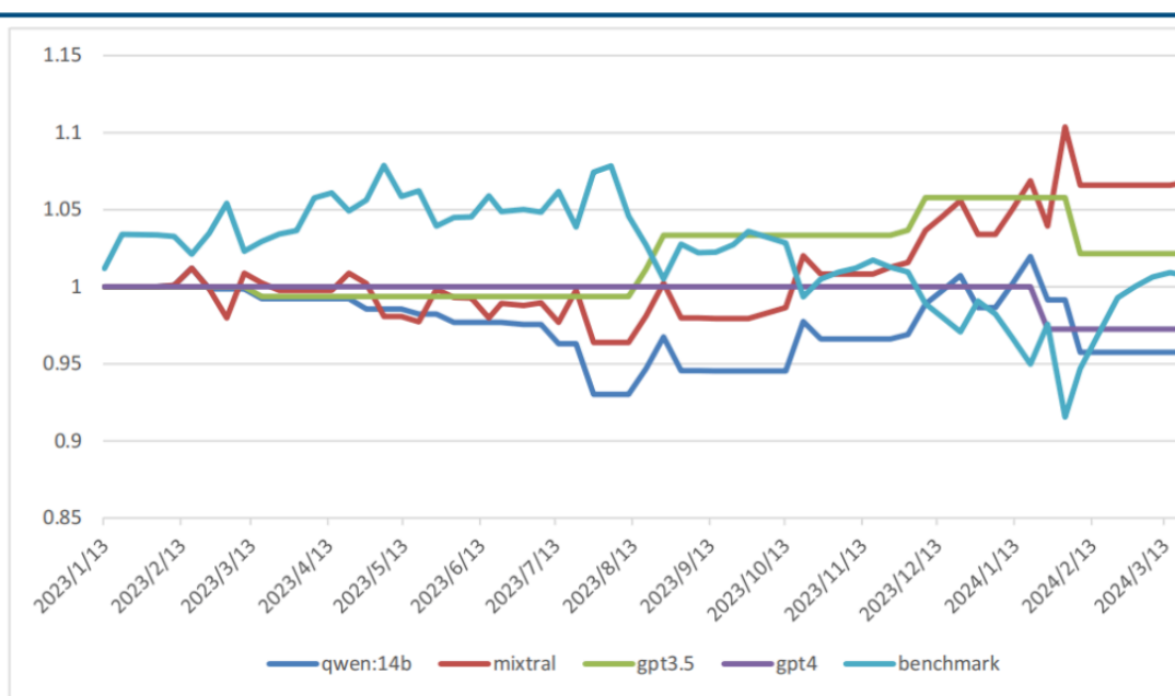
图 18: LLM 上证综指空头择时净值
