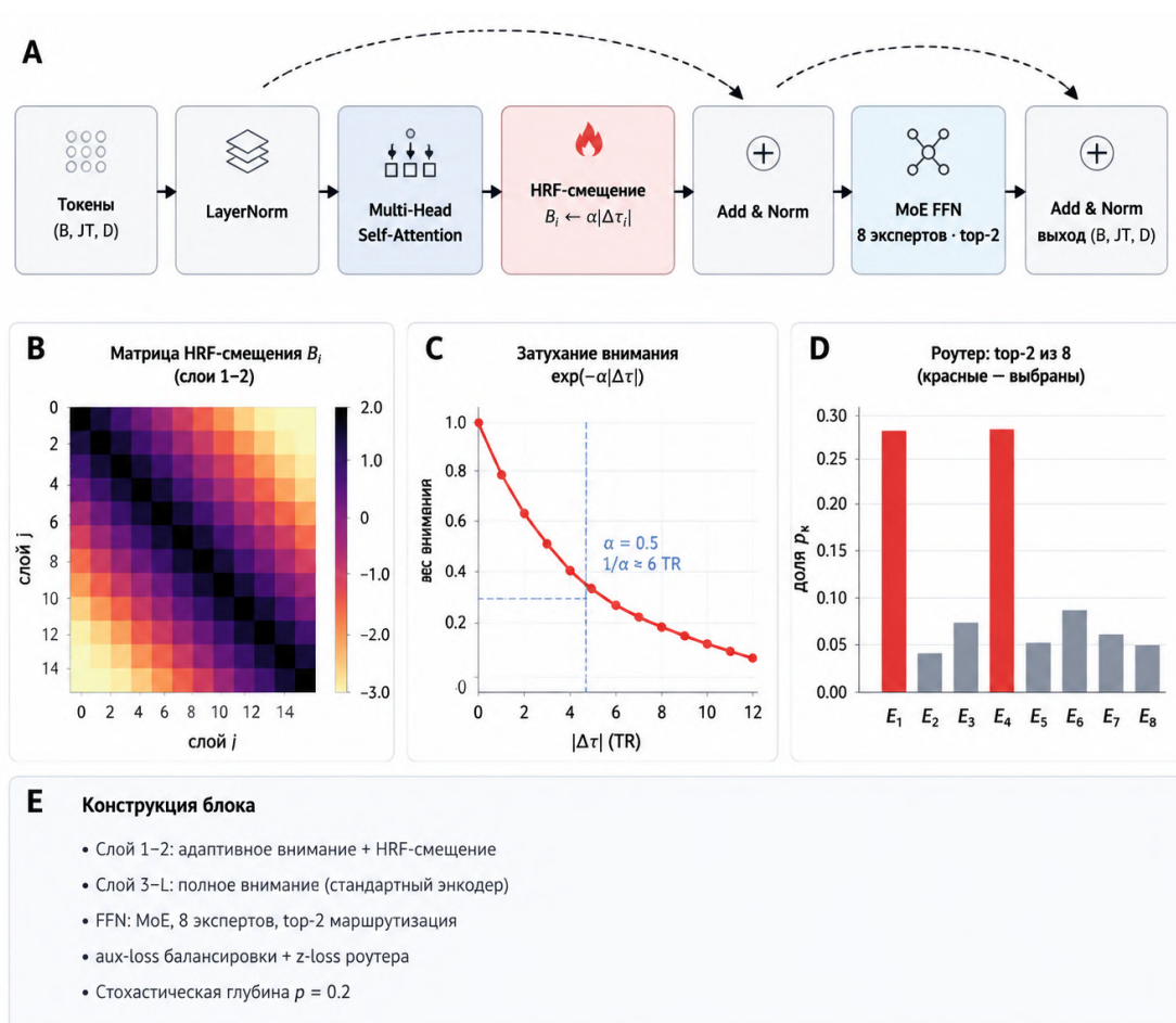
Рис. 4. Блок трансформера со смесью экспертов
