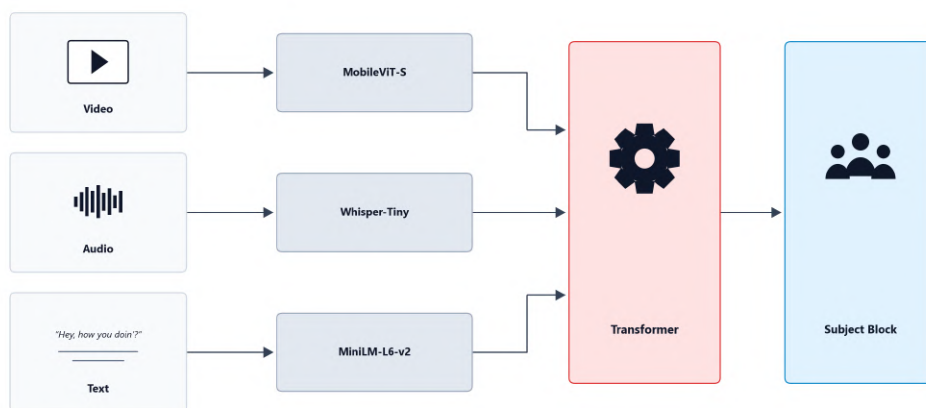
Рис. 3. Архитектура модели Flora
