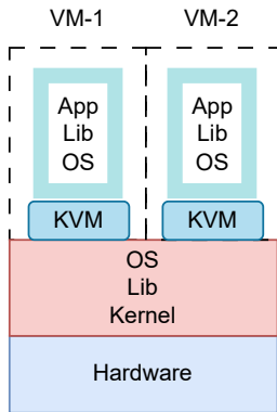
MicroVM
