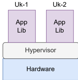
Unikernel
