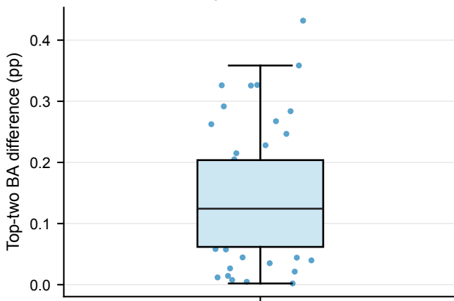
OrganAMNIST / A
