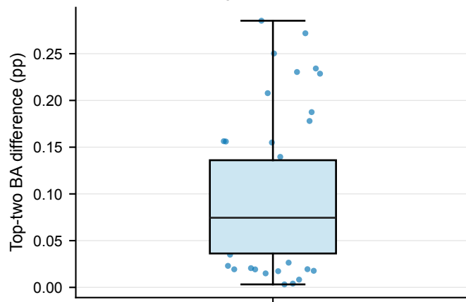
OrganAMNIST / B
