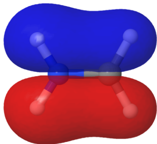
MO 5 (occ.) -1.041 E_h
