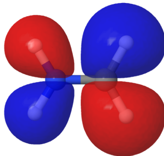
MO 7 (occ.) -0.845 E_h
