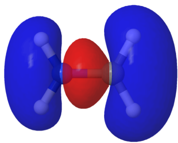
MO 6 (occ.) -0.974 E_h
