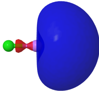
MO 11 (virt.) 0.003 E_h
