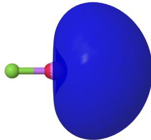
MO 7 (virt.) -0.001 E_h
