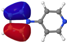
MO 38 (occ.) -0.315 E_h
