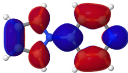
MO 39 (virt.) 0.102 E_h
