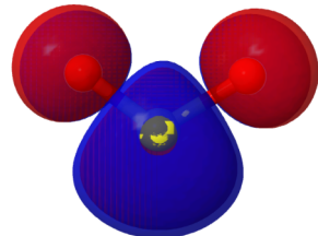
MO 17 (virt.) 0.014 E_h
