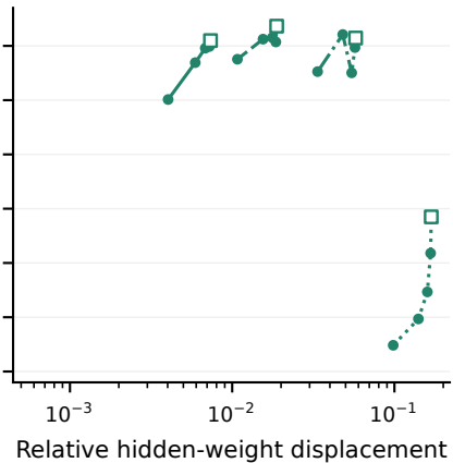
NorMuon
