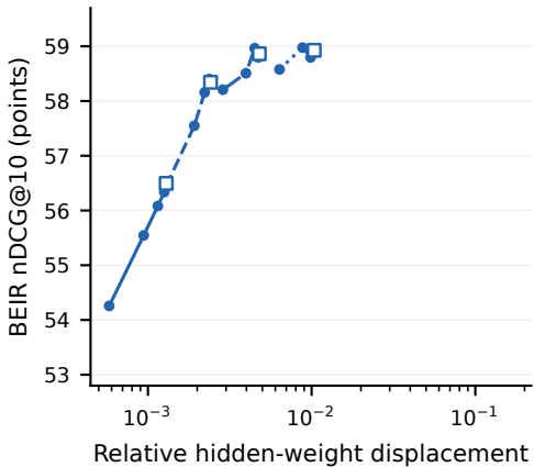
AdamW
