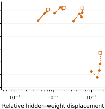
Muon
