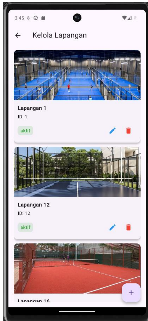
Tampilan index
