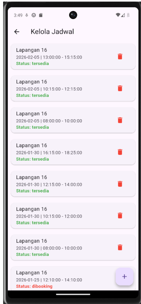
Tampilan index
