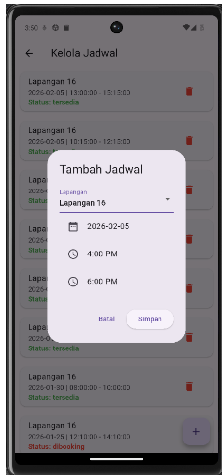
Form tambah
