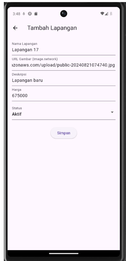
Form tambah
