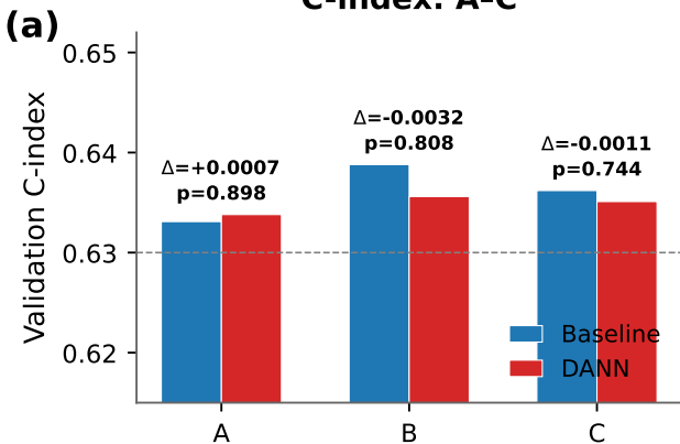
C-index: A-C
