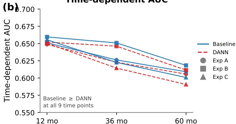
Time-dependent AUC
