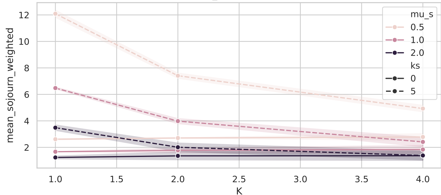
E[T] vs K ( \lambda=4.0 , \mu_f=2.0 , backup systématique)
