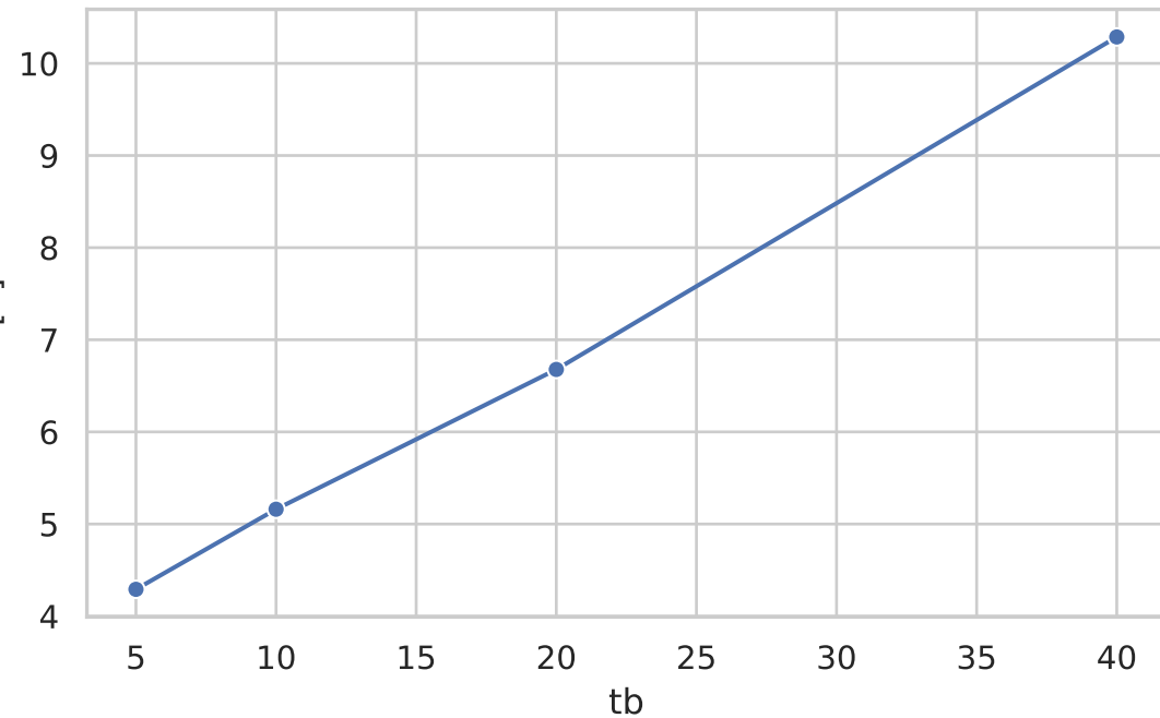
ING — E[T] vs tb (barrage FIFO)
