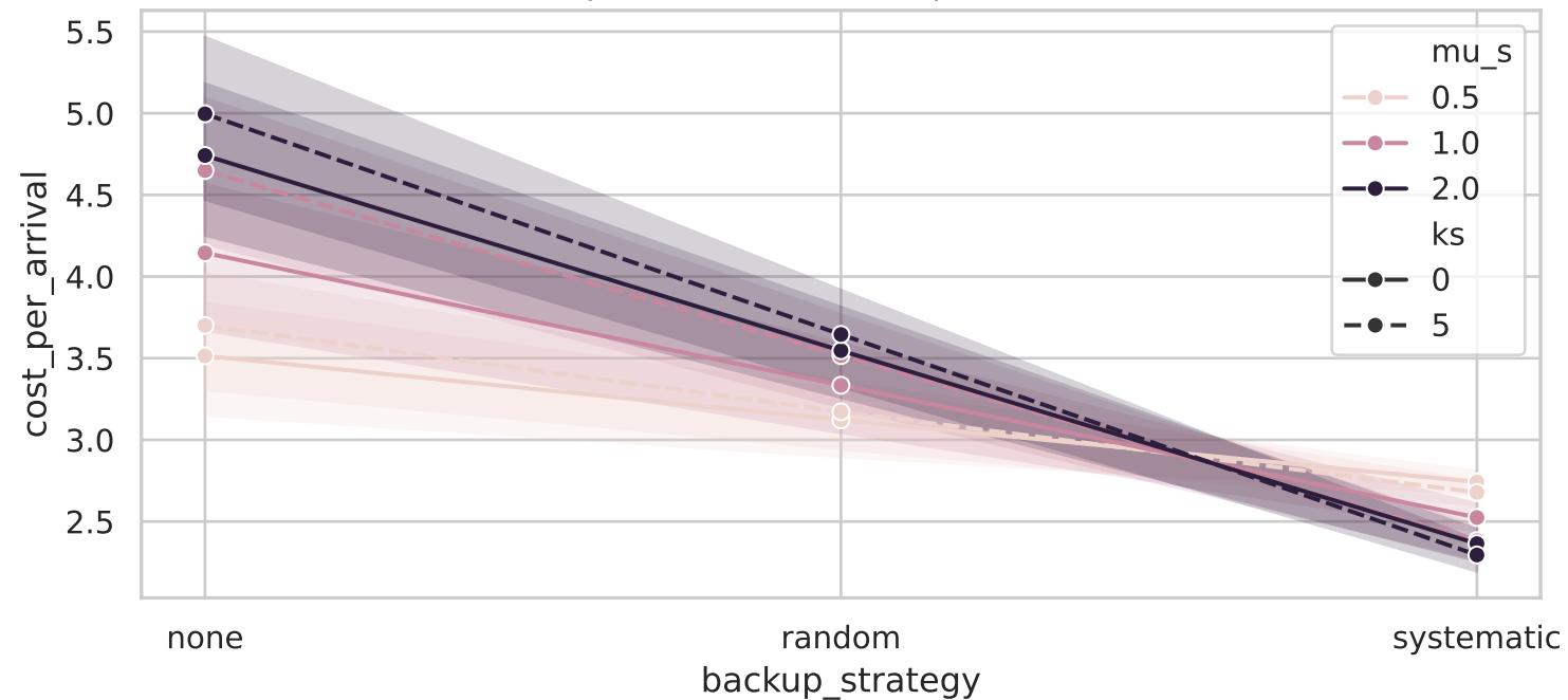
Coût par arrivée vs backup ( \lambda=4.0 , K=4 )
