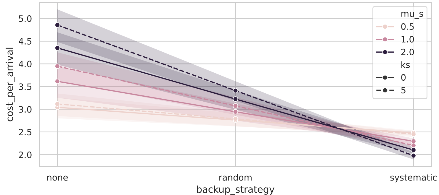
Coût par arrivée vs backup ( \lambda=6.0 , K=4 )
