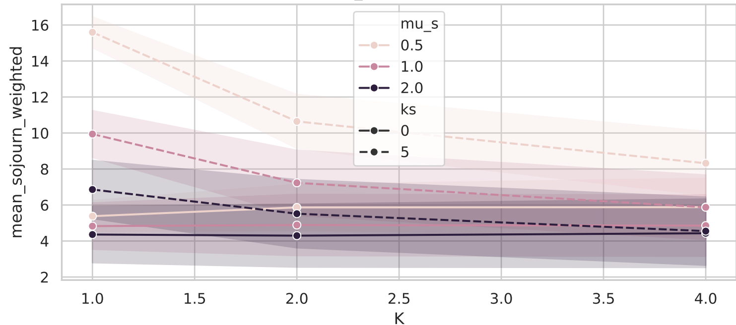
E[T] vs K ( \lambda=6.0 , \mu_f=0.5 , backup systématique)
