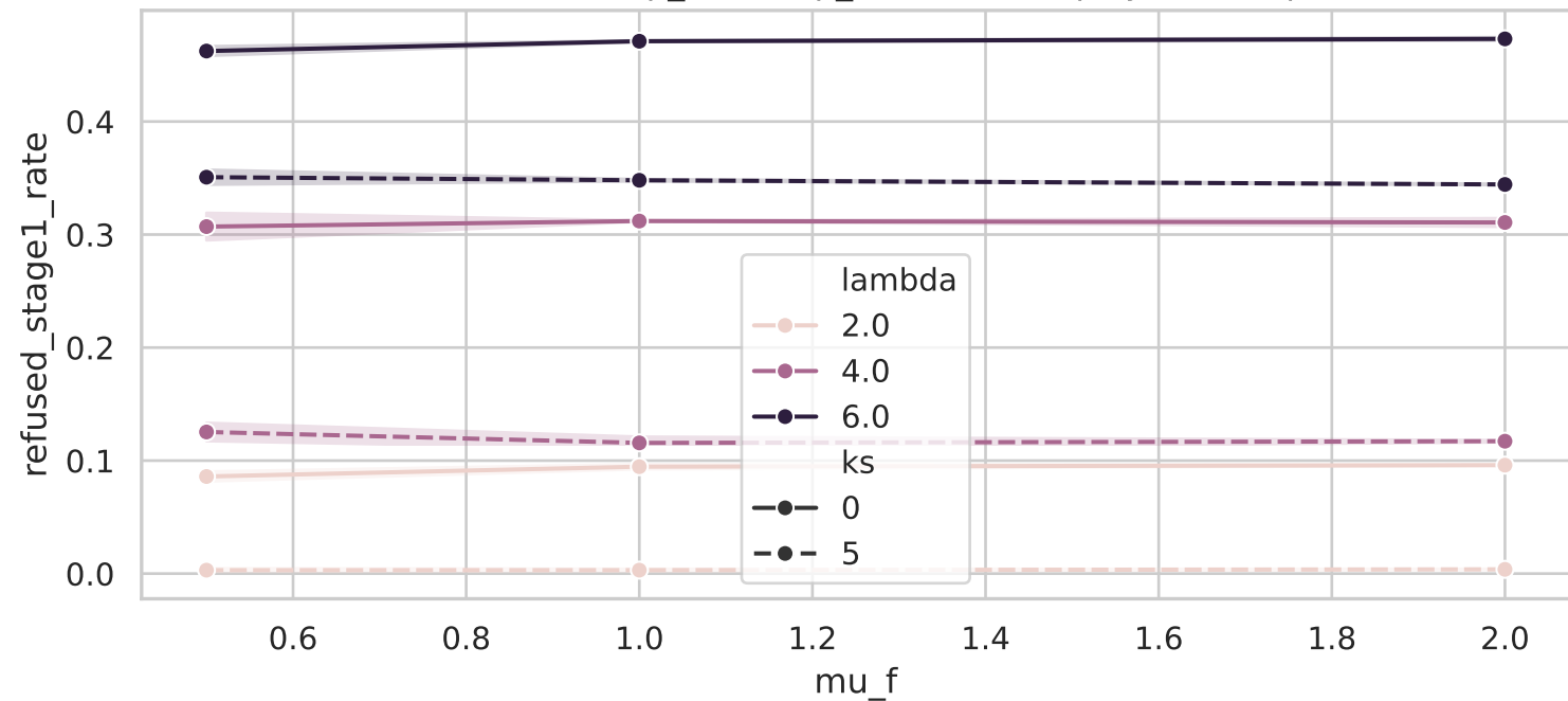
Taux de refus vs \mu_f ( K=4 , \mu_s=1.0 , backup systématique)
