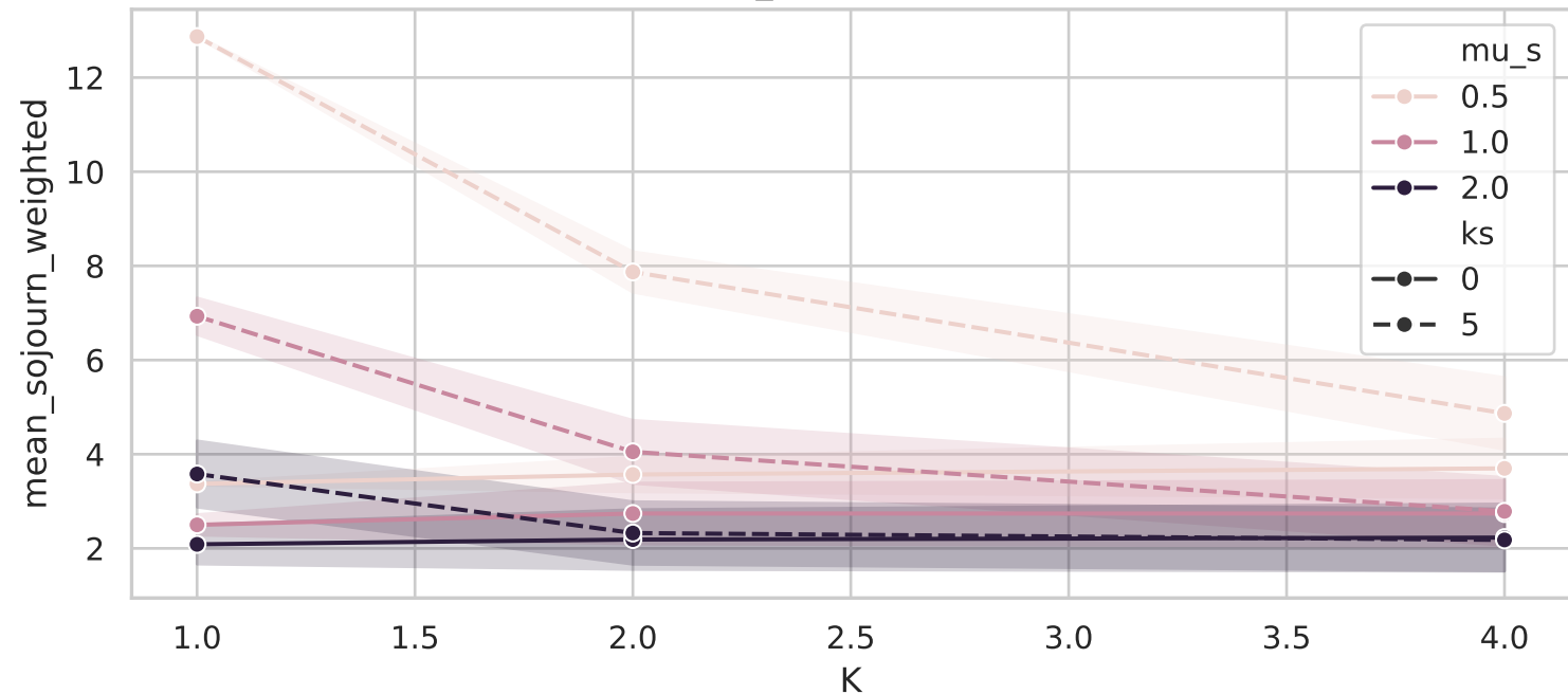
E[T] vs K ( \lambda=2.0 , \mu_f=1.0 , backup systématique)
