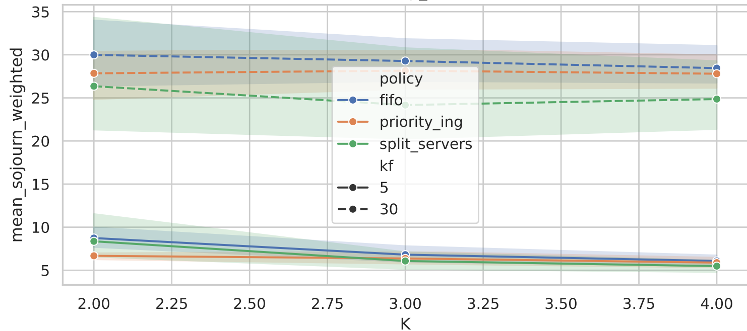
ING — E[T] vs K ( \mu_f=1.0 , ks=10 )
