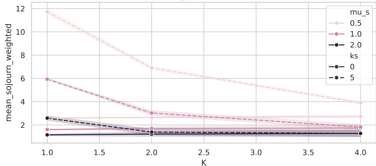
E[T] vs K ( \lambda=2.0 , \mu_f=2.0 , backup systématique)
