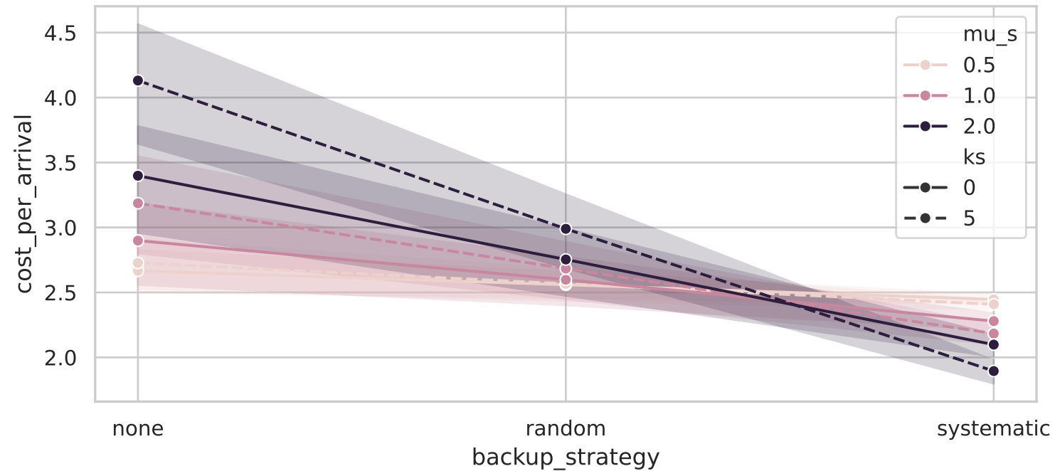
Coût par arrivée vs backup ( \lambda=4.0 , K=2 )
