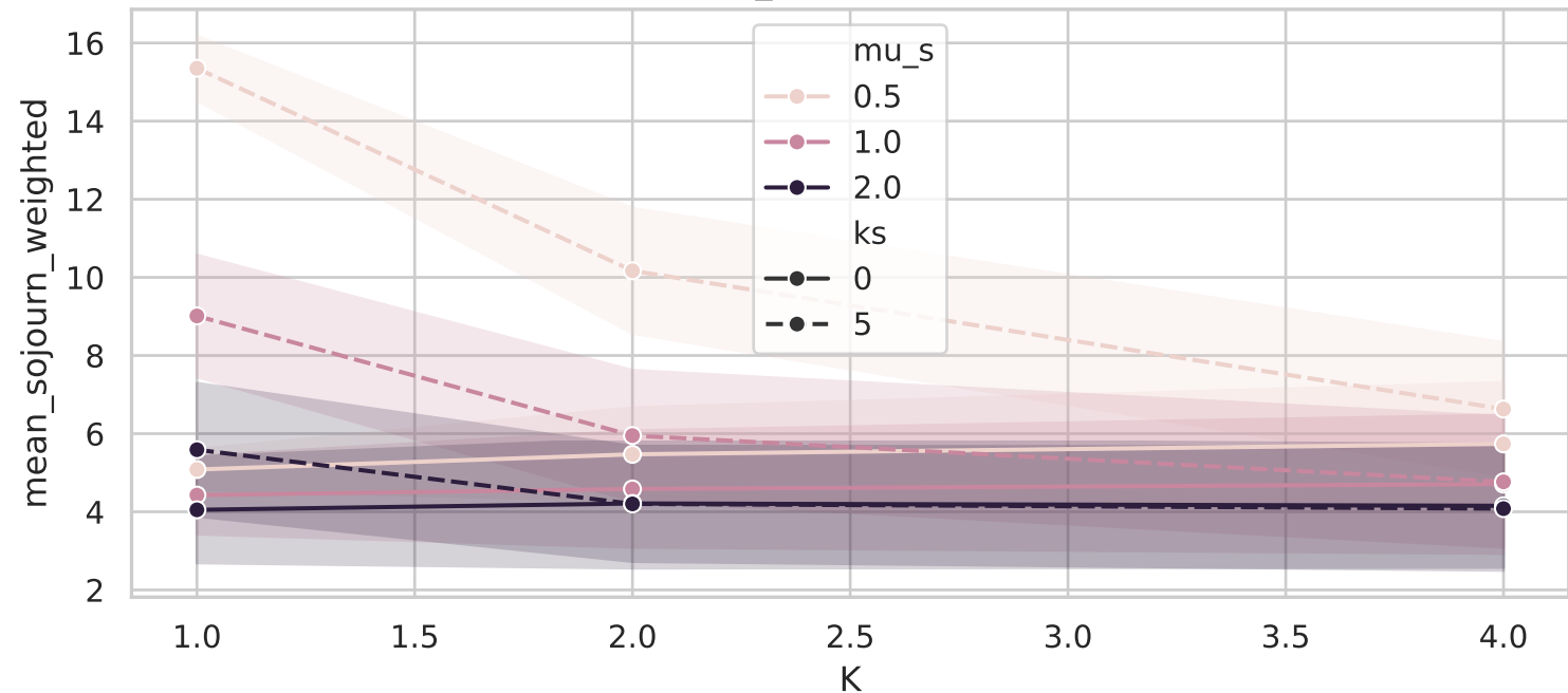
E[T] vs K ( \lambda=2.0 , \mu_f=0.5 , backup systématique)
