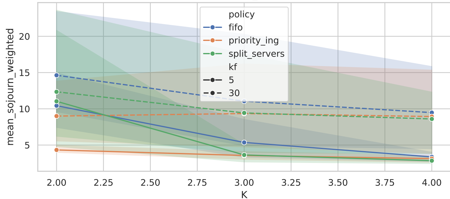
ING — E[T] vs K ( \mu_f=2.0 , ks=30 )
