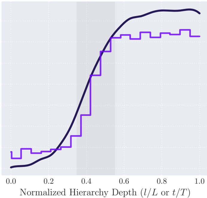
CelebA
