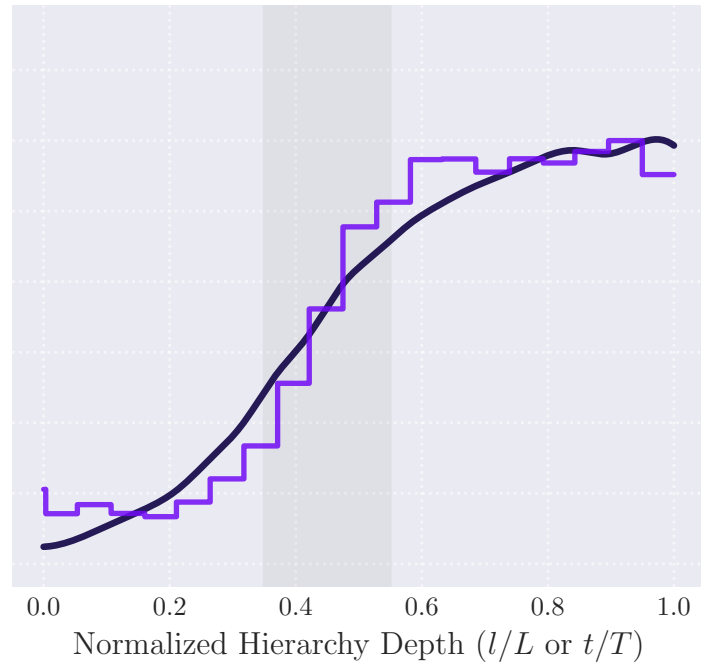
ImageNet-32
