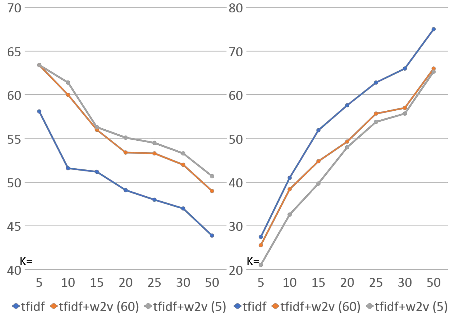
Precision
