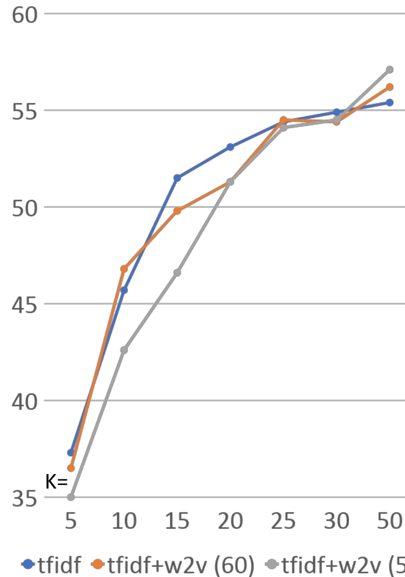
F1
