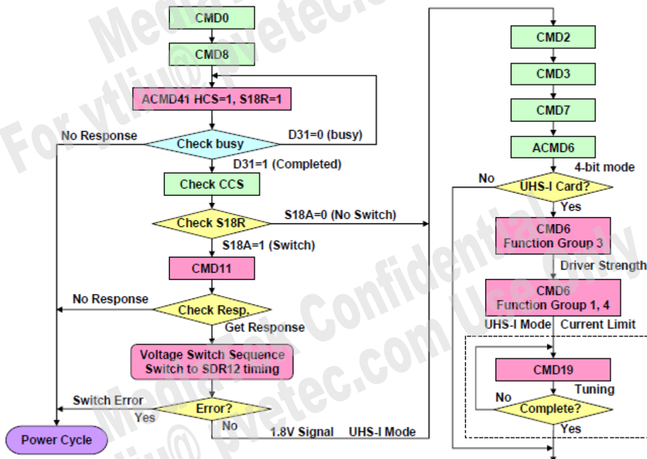
图 1-1. UHS-I 卡初始化流程
