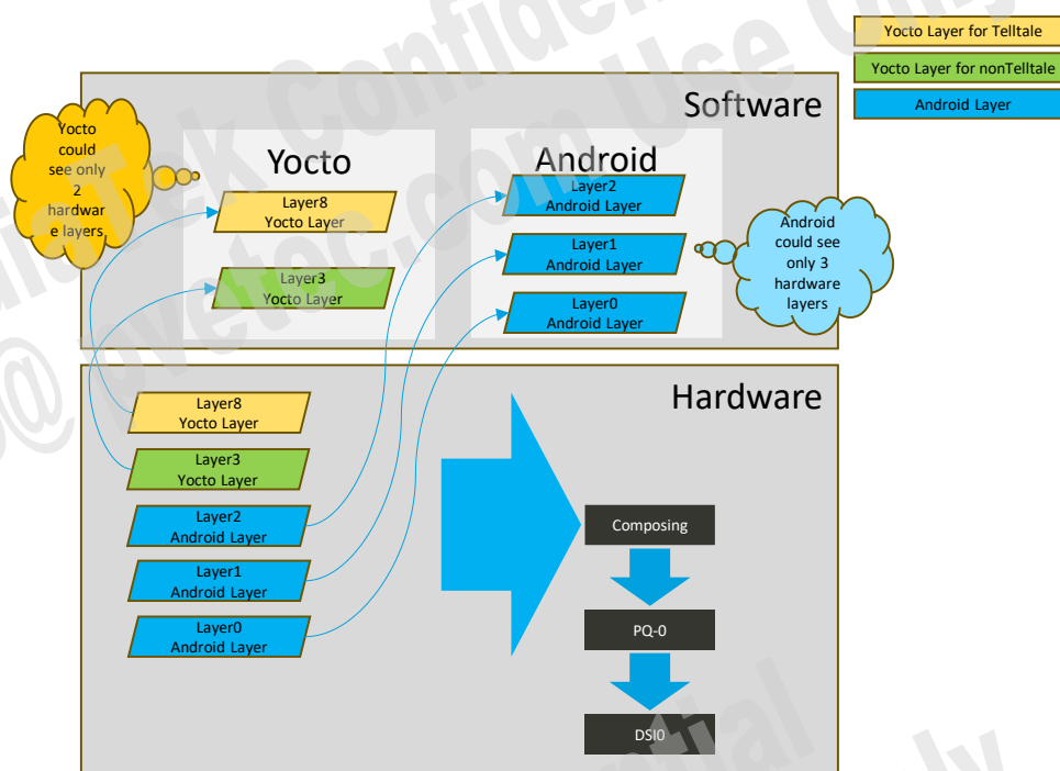
图 1-4. exDMA Config on Pipeline-0 示例
