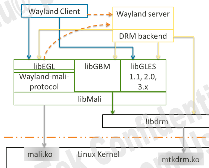
图 1-1. Yocto 图形框架
