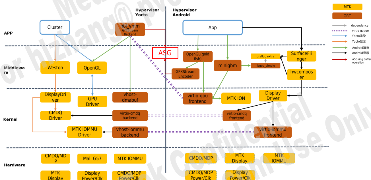
图 1-1. Hypervisor 图形框架
