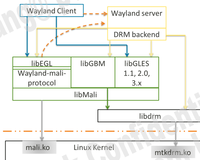
图 1-1. Yocto 图形框架
