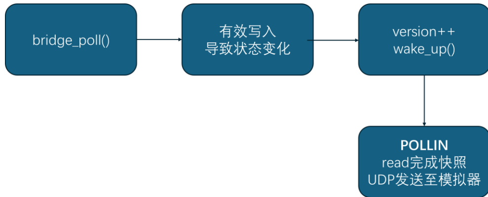
图 3 wait queue 与 poll 事件路径
