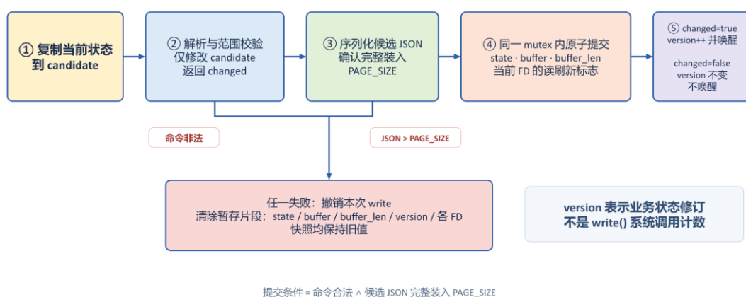
图 5 write() 候选状态事务
