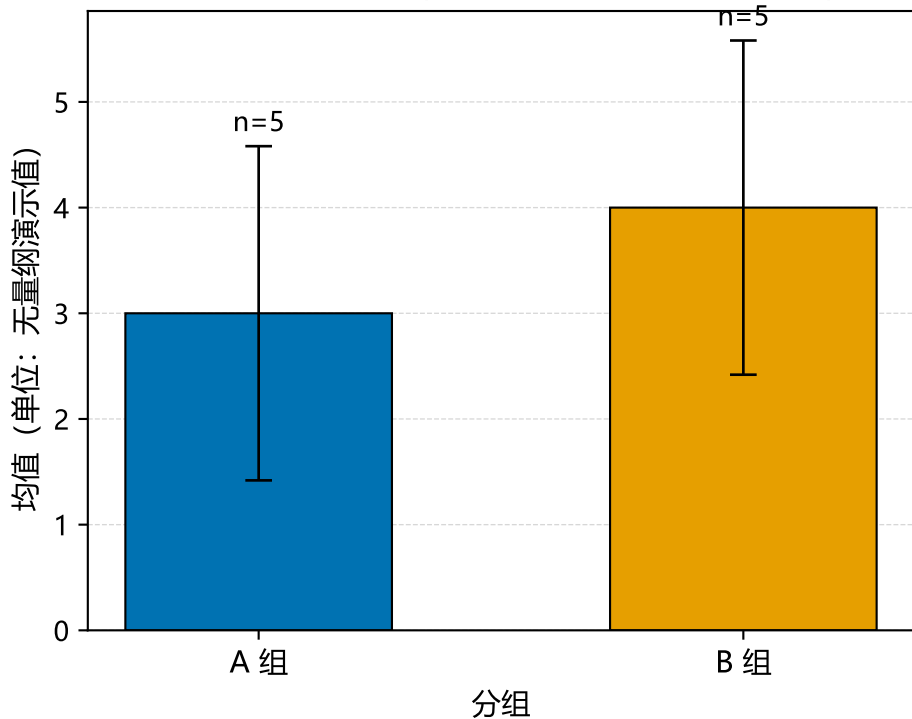
A、B 两组均值对比 (误差条 = 样本标准差, ddof=1)
