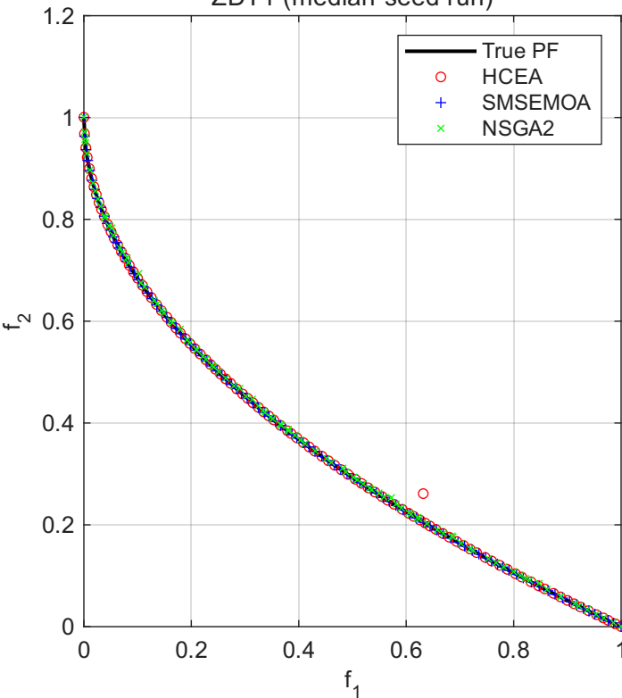
ZDT1 (median-seed run)
