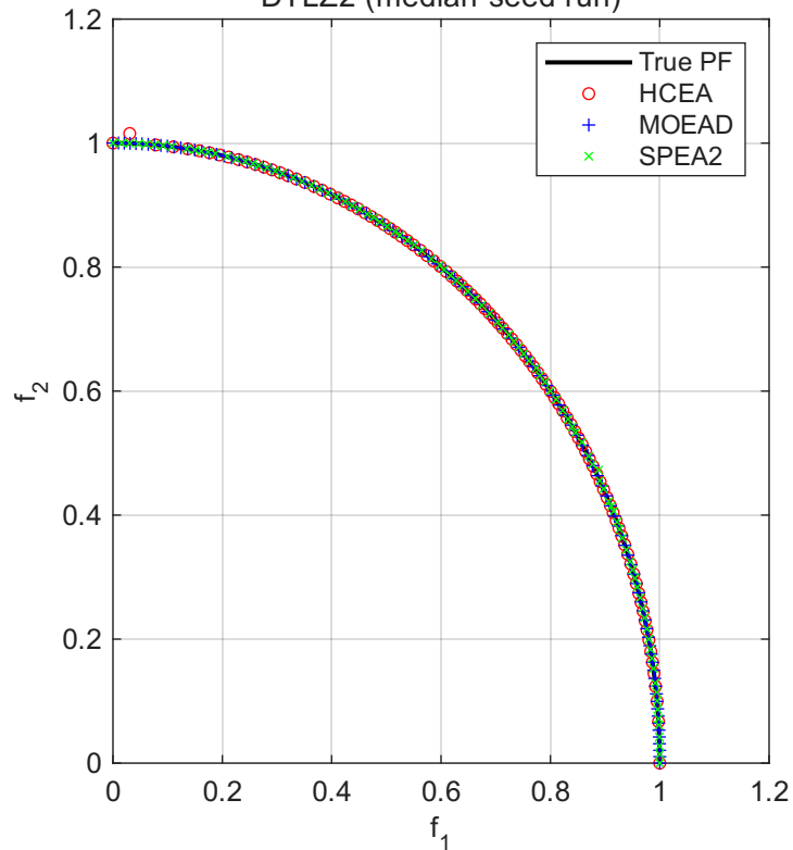
DTLZ2 (median-seed run)
