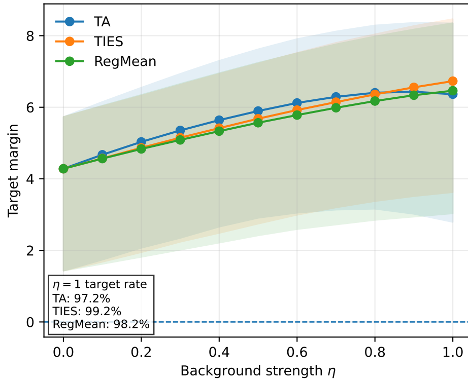
(b) BadMerging-On
