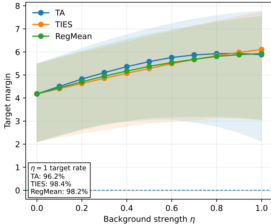
(b) BadMerging-On
