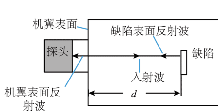
图 (a) 超声波检测原理示意图
