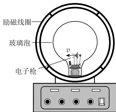
图甲 洛伦兹力演示仪示意图
