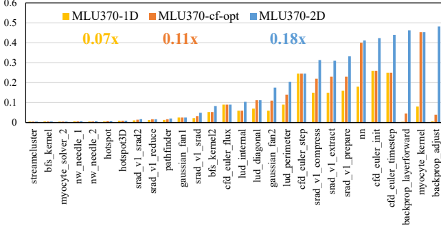
(b) MLU370
