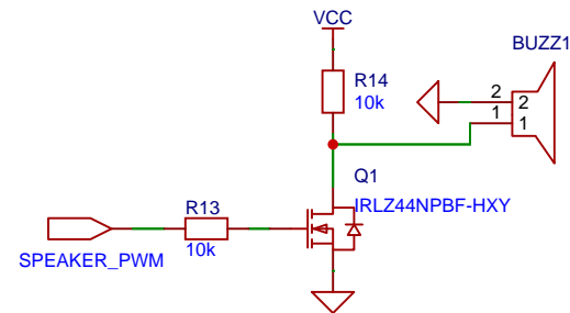
扬声器
