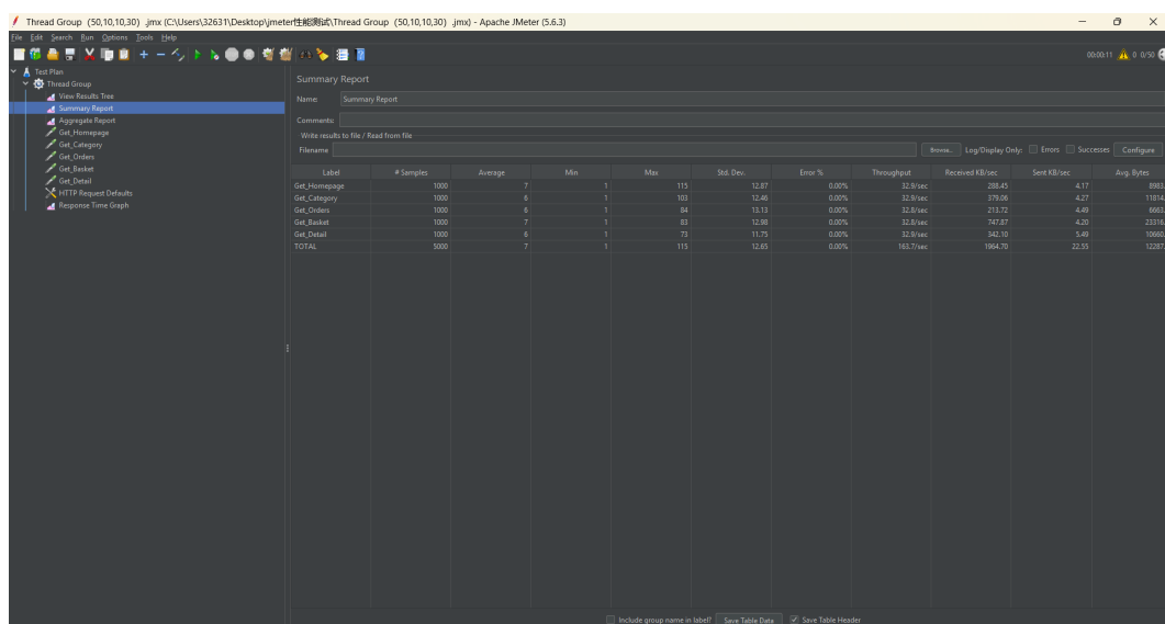
图 10: Scene-2 (50 并发) 汇总报告
