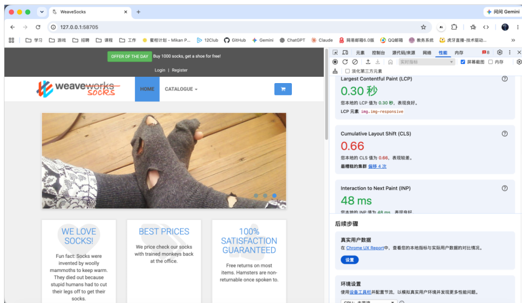
图 5: Chrome DevTools 性能指标测试截图
