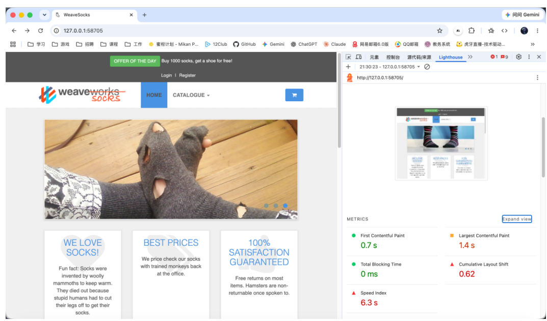
图 6: Lighthouse 性能评测结果截图
