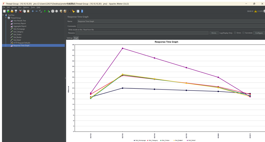
图 9: Scene-1 (10 并发) 响应时间图
