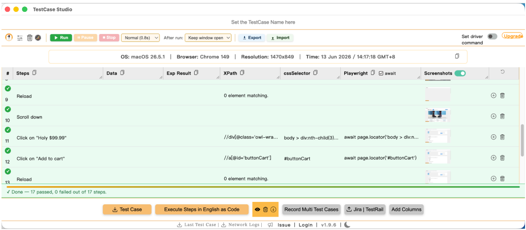
图 4: Chrome 浏览器 Testcase Studio 插件测试截图
