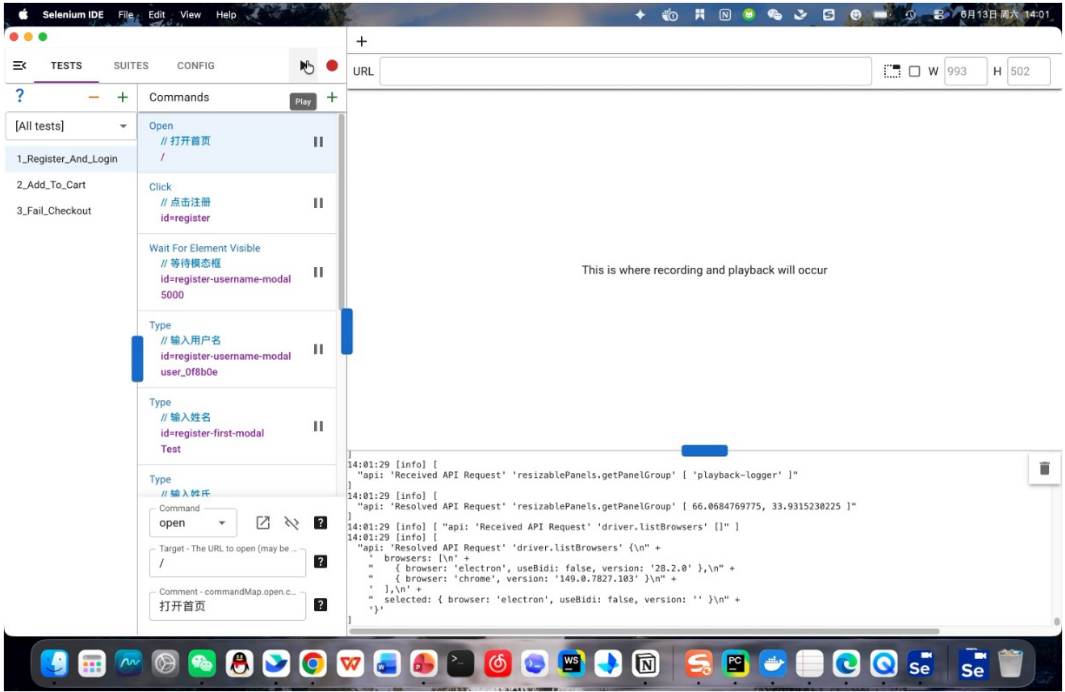
图 3: Selenium IDE 前端功能测试截图（注册、登录、购物及结算流程）
