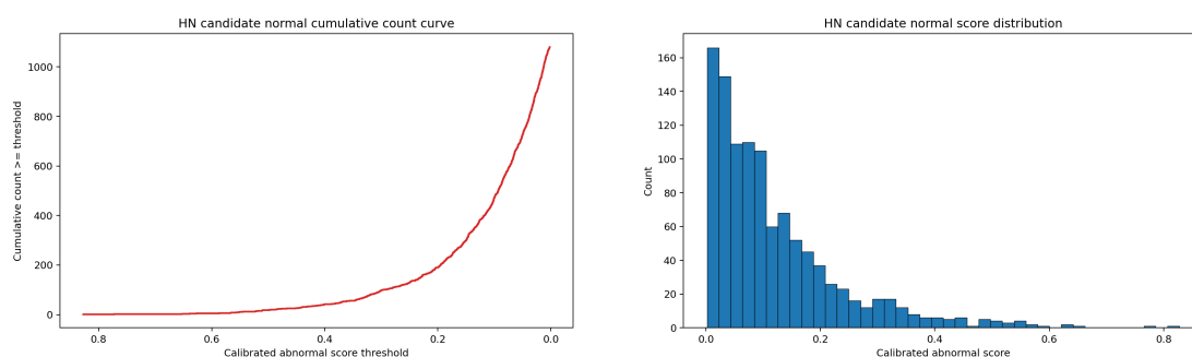
图 4 第一阶段 HN 候选样本累计数量与分数分布补充图
