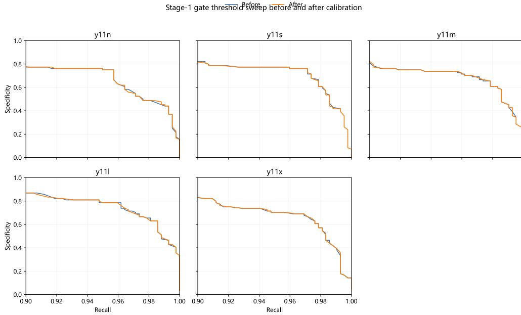
图 4.3 五模型 Calibration 前后 threshold sweep 对比
