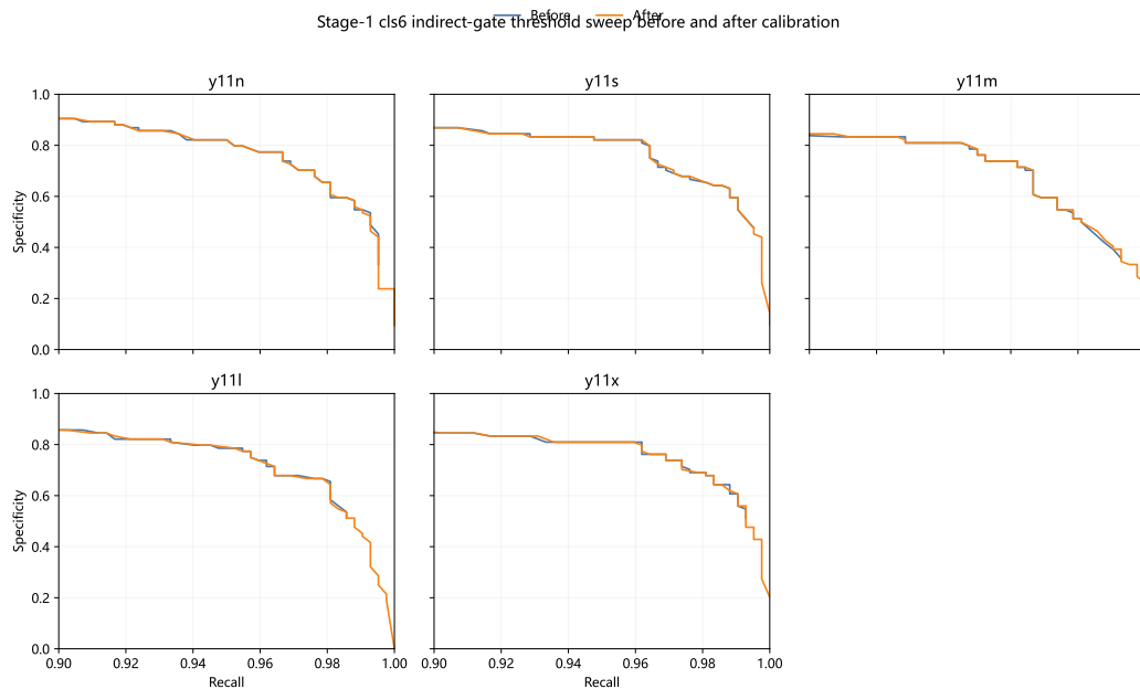
图 2 六类间接 gate 五模型的 calibration 前后 threshold sweep 对比
