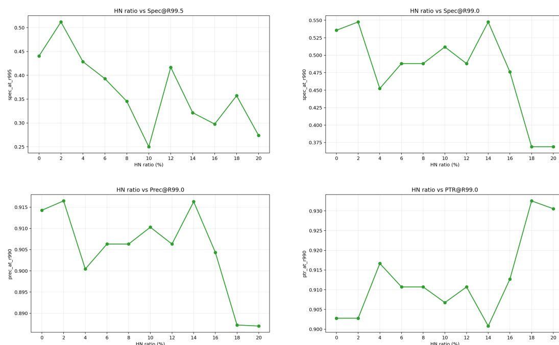
图 4.4 第一阶段 HN 回流比例扫描关键指标对比
