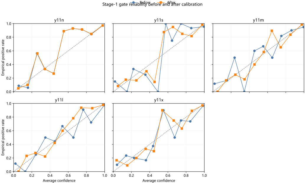
图 4.2 五模型 Calibration 前后 Reliability Diagram 对比
