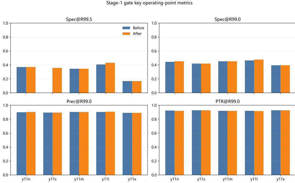
图 4.1 第一阶段不同模型容量的关键指标对比
