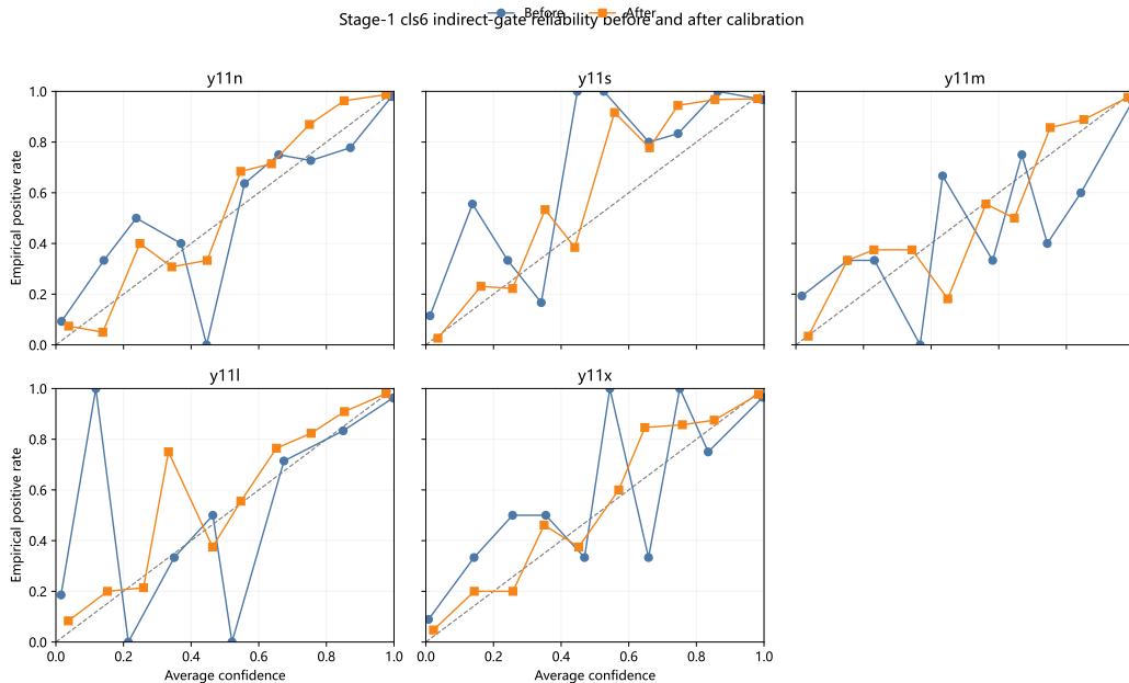
图 1 六类间接 gate 五模型的 Reliability Diagram 对比
