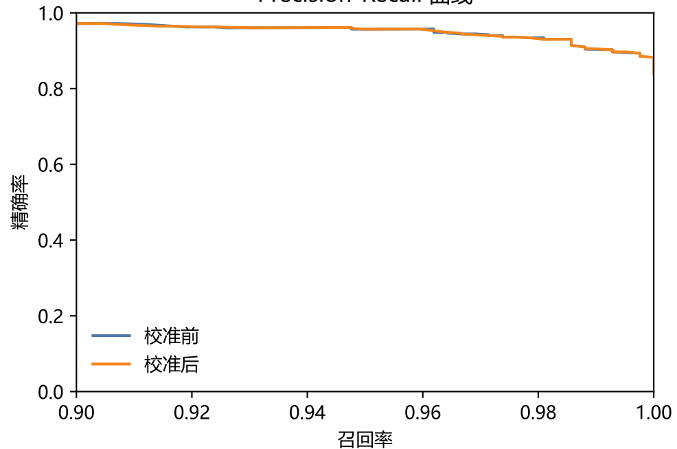
Precision-Recall 曲线
