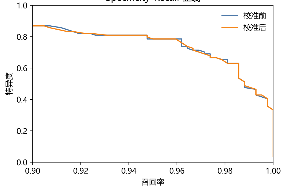
Specificity-Recall 曲线
